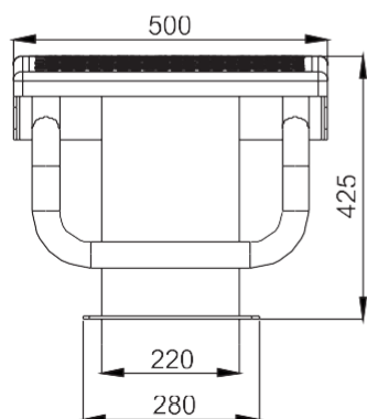
Platforma startowa (jednostka miary: mm)
