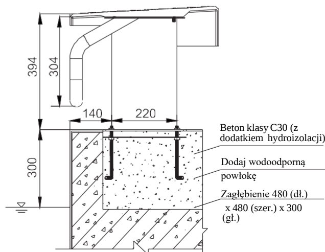
Schemat montażu (Jednostka miary: mm)
